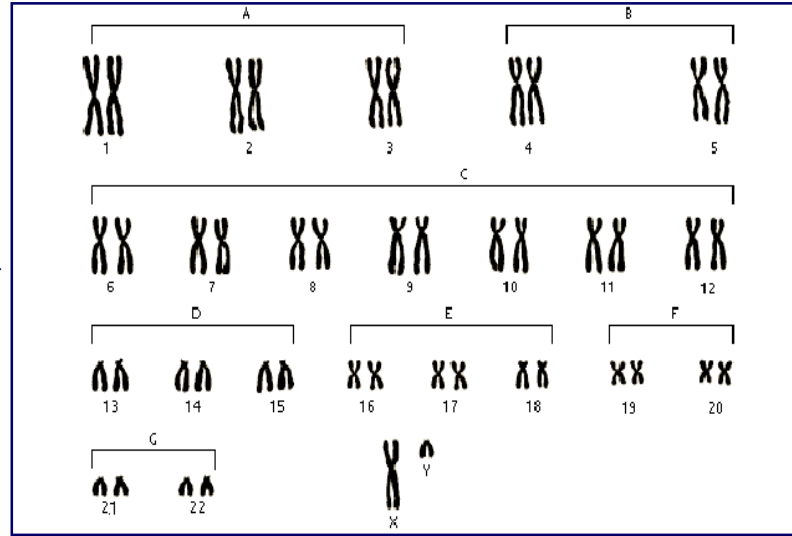
Karyotip
