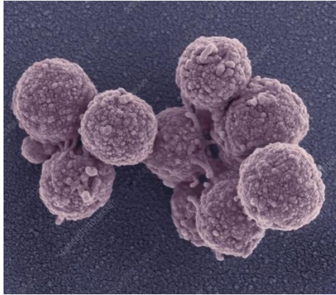
M. genitalium
