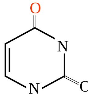
URASİL
