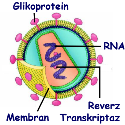
AIDS Virüsü
