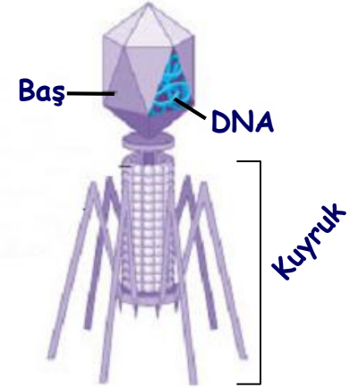
T2/T4 Bakteriyofaj
