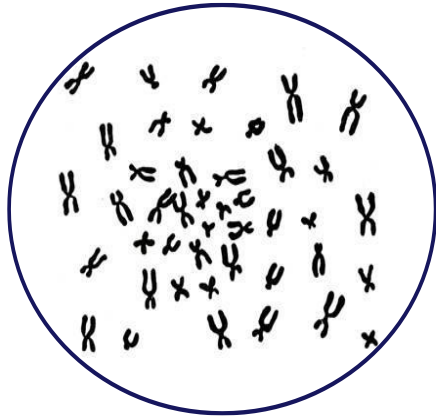
Karyotip
