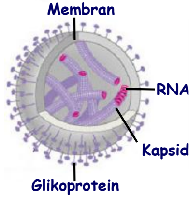
İnfluenza Virüsü
